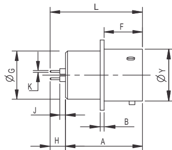
Style 12E(220) Im wire terminations
