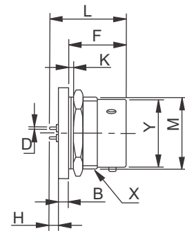
Style 57A(219) Im wire terminators
